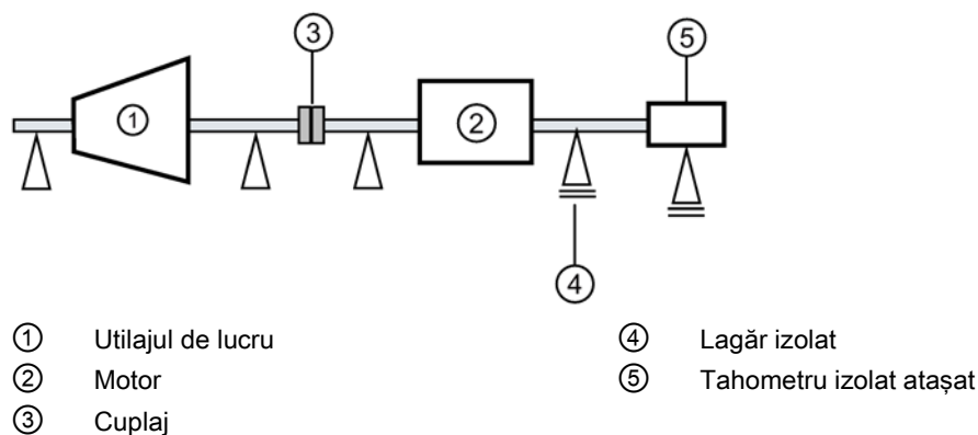
Imagine 4-2 Reprezentare de principiu a acționării individuale
