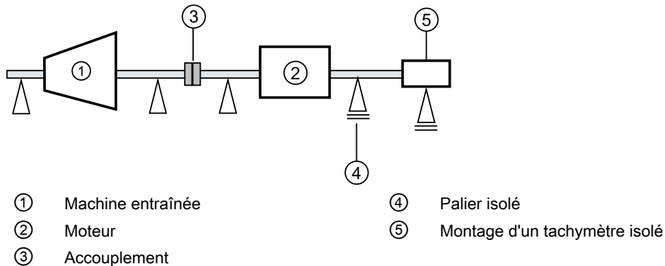
Figure 4-2 Schéma de principe de l'entraînement monomoteur
