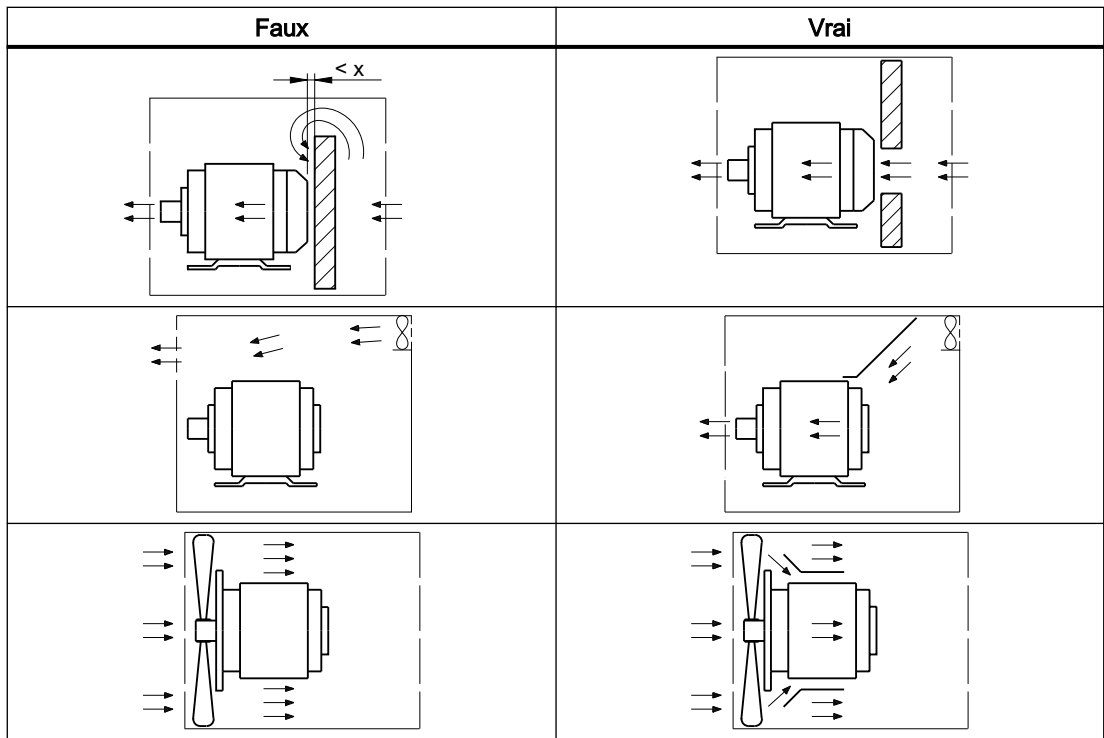
Cote minimale "x" pour l'écart entre modules voisins pour l'entrée d'air de la machine
