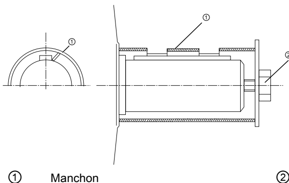
Figure 4-1 Fixation axiale du rotor
