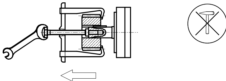
Retrait des organes de transmission
